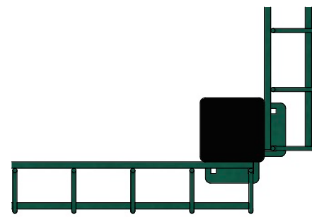
EXTERNAL CORNER POST scale: 1:5
